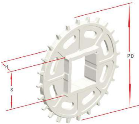
Sprocket Dimensions
